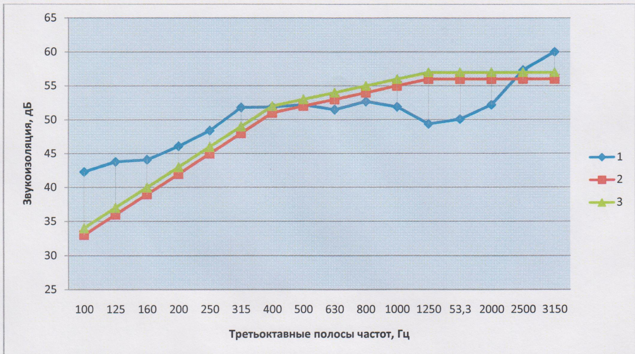
Рисунок 1. Частотная характеристика звукоизоляции
